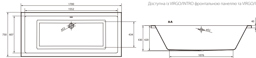
INTRO 170 прямокутна ванна INTRO 170 прямоугольная ванна
