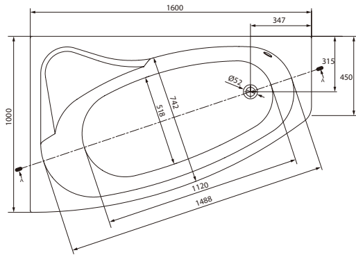
SICILIA 160 асиметрична ванна ліва/права SICILIA 160 асимметричная ванна левая/правая
